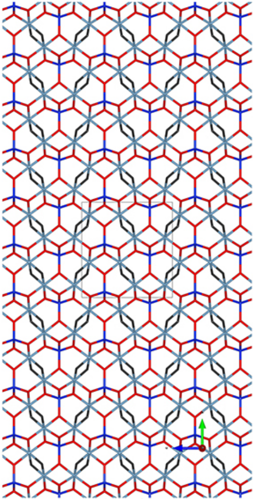
a-Stick-Mol.jpg
