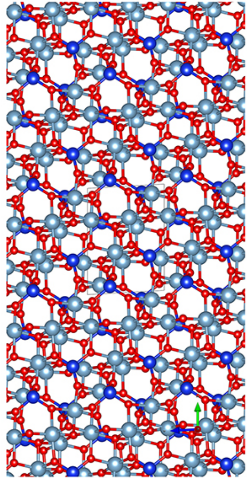
a-Ball&Stick-Mol.jpg
