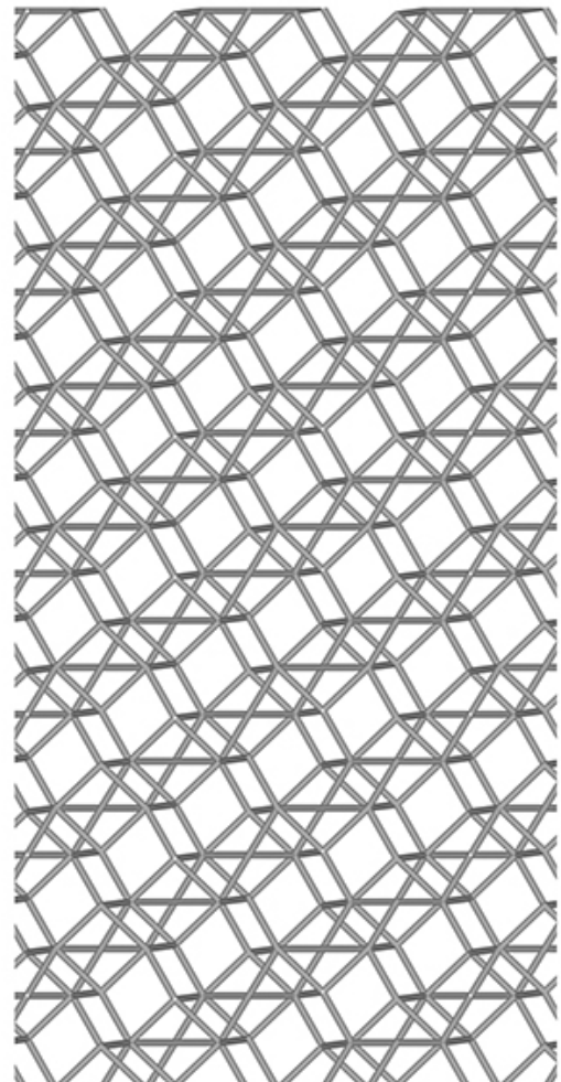
a-Stick-Mol-U.jpg
