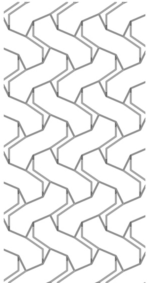
a-Stick-Mol-U.jpg
