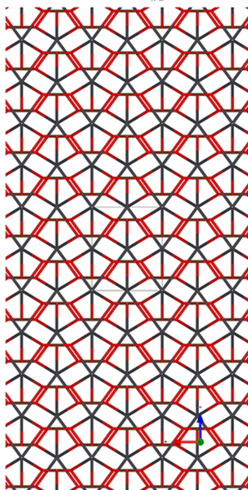
b-Stick-Mol.jpg
