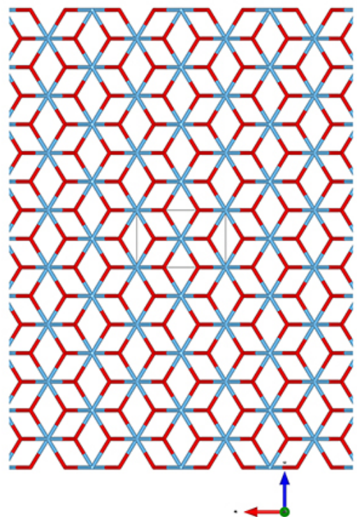
b-Stick-Mol.jpg
