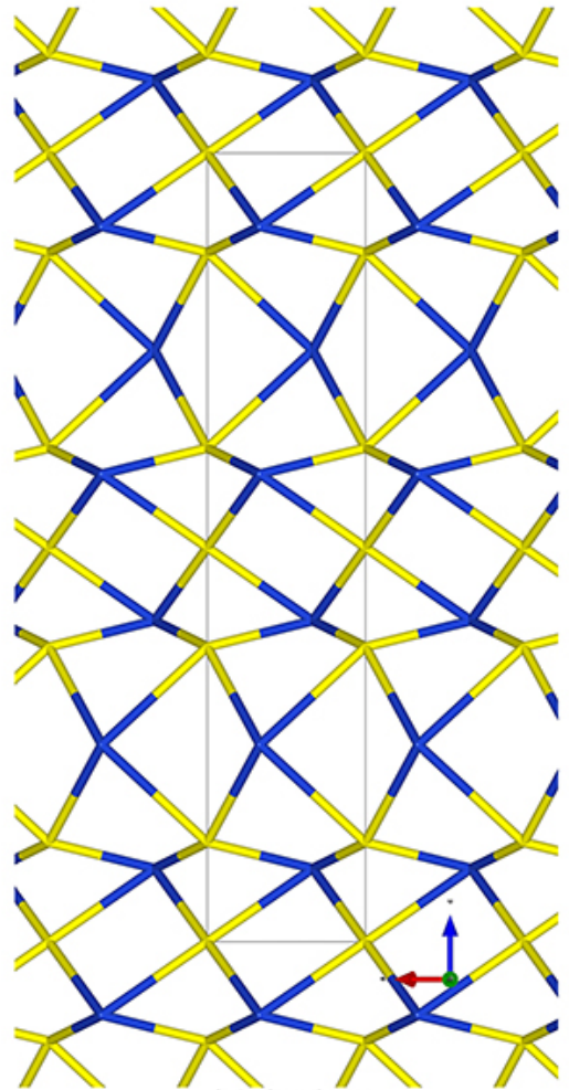
b-Stick-Mol.jpg
