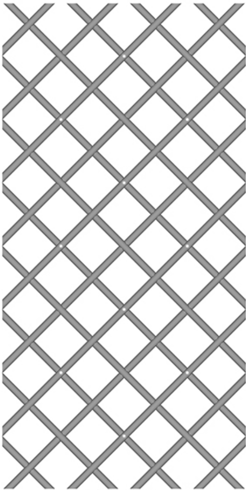
a-Stick-Mol-U.jpg
