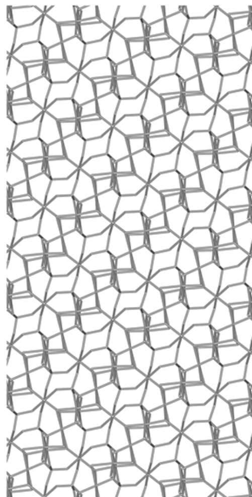
b-Stick-Mol-U.jpg
