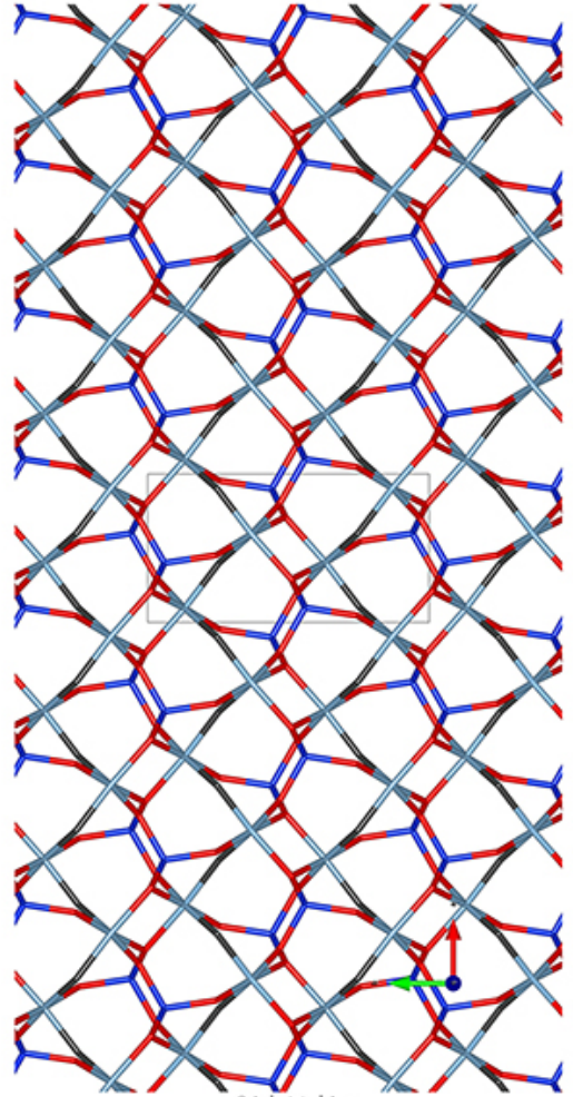
c-Stick-Mol.jpg
