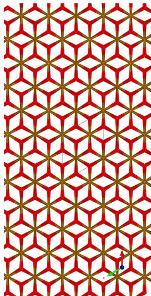
c-Stick-Mol.jpg
