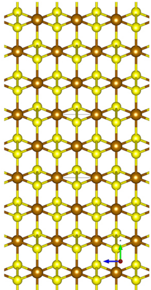
a-Ball&Stick-Mol.jpg
