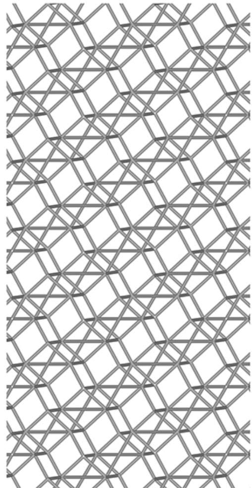
a-Stick-Mol-U.jpg
