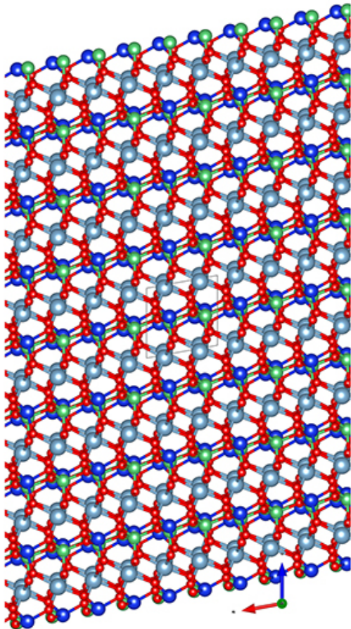
b-Ball&Stick-Mol.jpg
