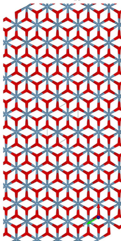
c-Stick-Mol.jpg
