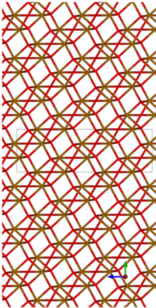
a-Stick-Mol.jpg
