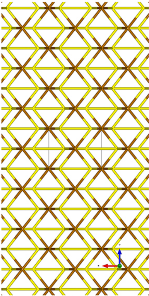
b-Stick-Mol.jpg
