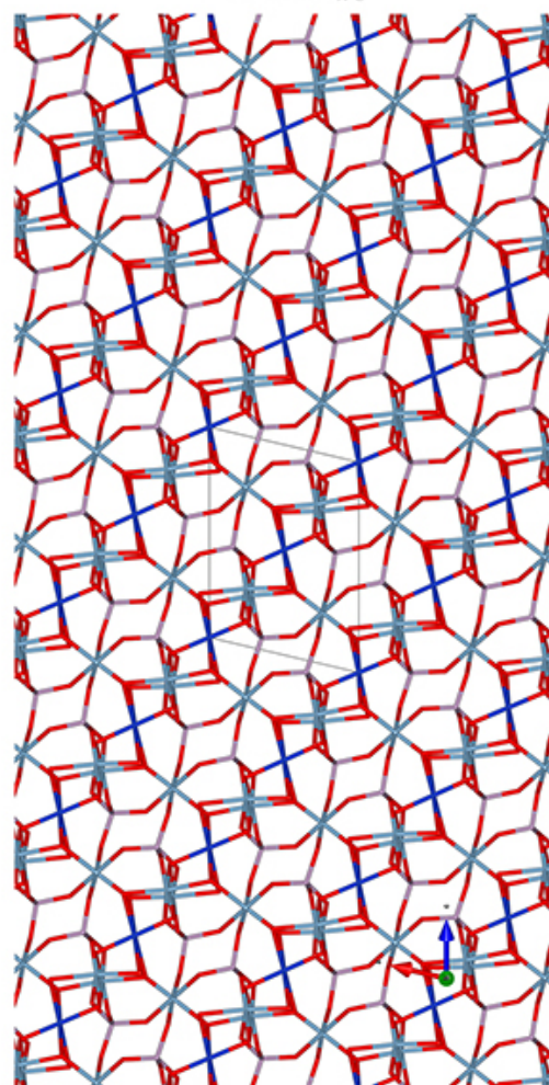
b-Stick-Mol.jpg
