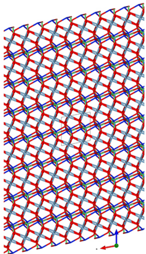
b-Stick-Mol-U.jpg
