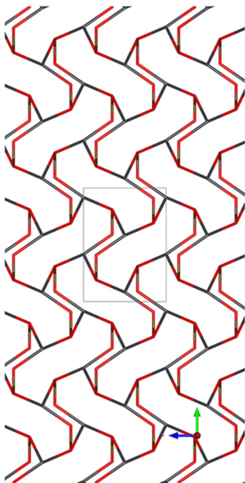
a-Stick-Mol.jpg
