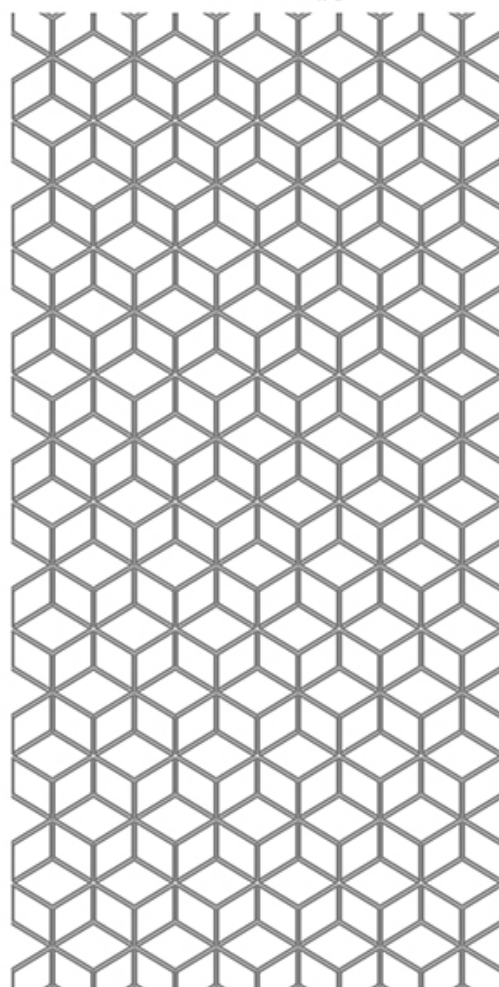
a-Stick-Mol-U.jpg
