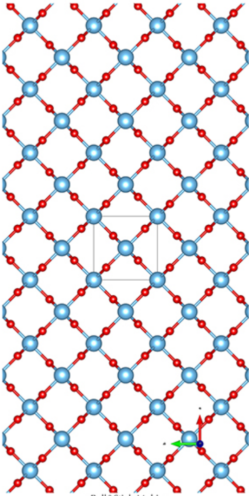
c-Ball&Stick-Mol.jpg
