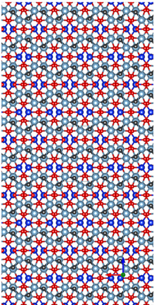
b-Ball&Stick-Mol.jpg
