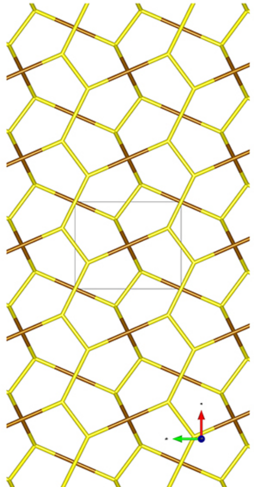
c-Stick-Mol.jpg
