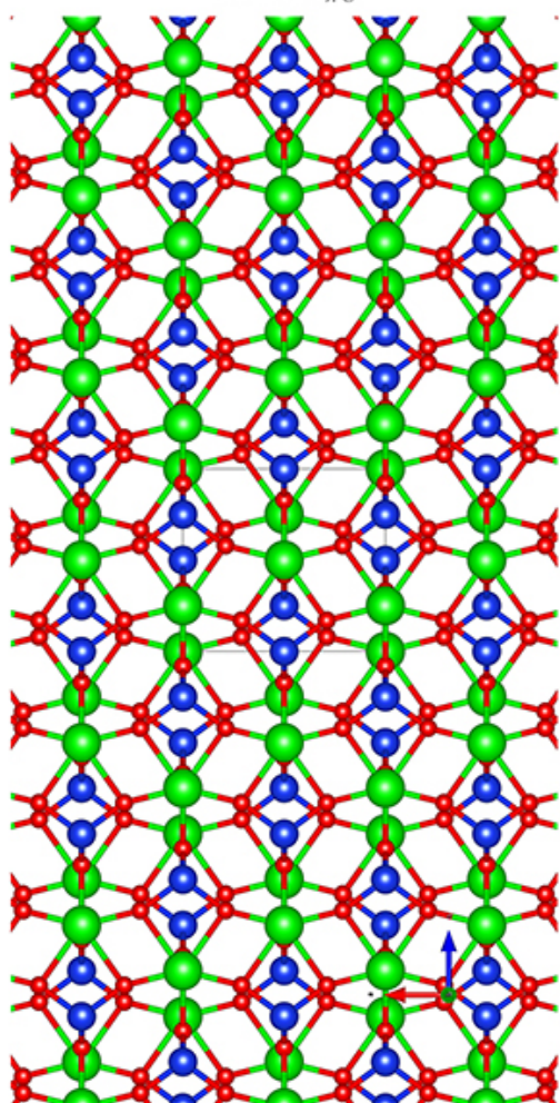
b-Ball&Stick-Mol.jpg
