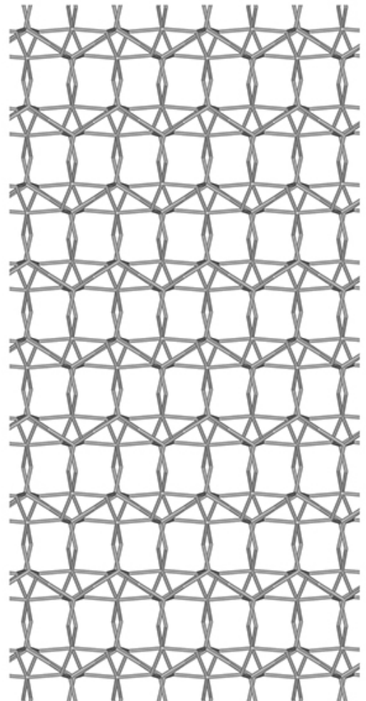
a-Stick-Mol-U.jpg
