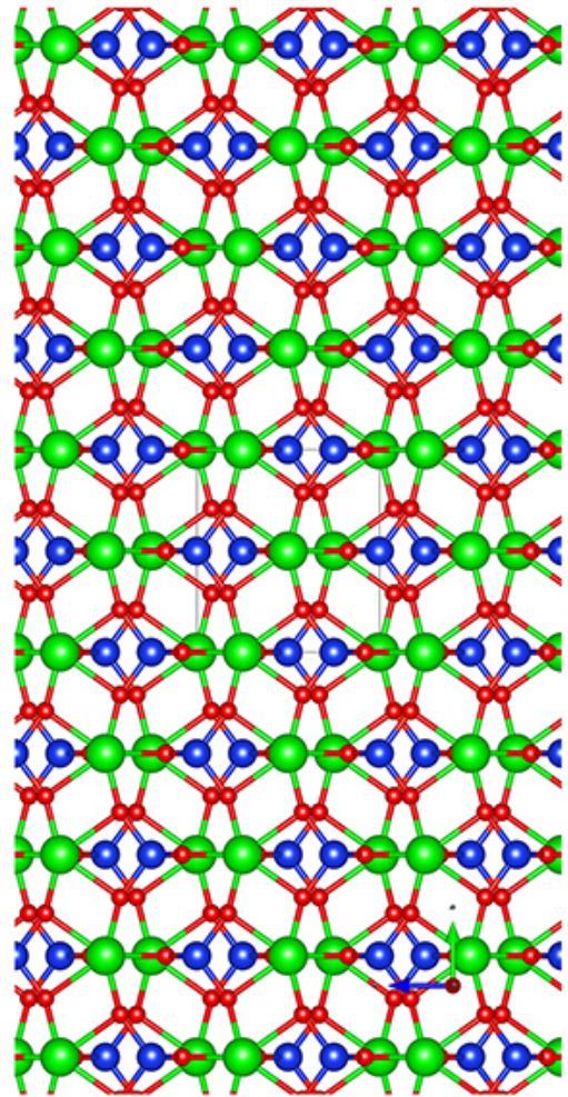
a-Ball&Stick-Mol.jpg
