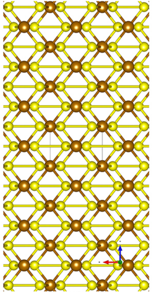
b-Ball&Stick-Mol.jpg
