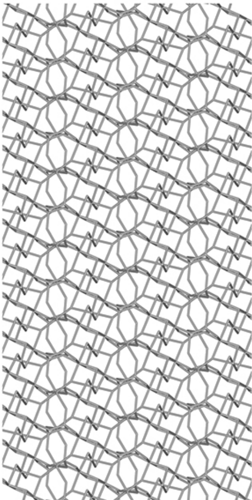
c-Stick-Mol-U.jpg
