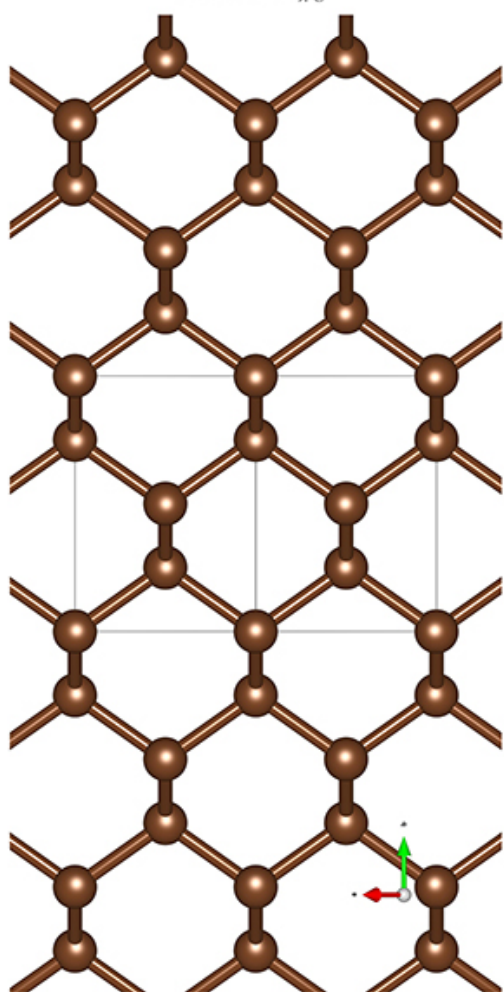
a3-Ball&Stick-Mol.jpg
