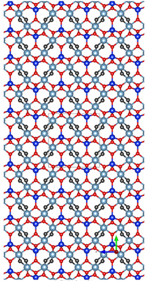
a-Ball&Stick-Mol.jpg
