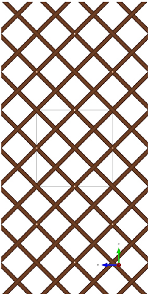
a-Stick-Mol.jpg
