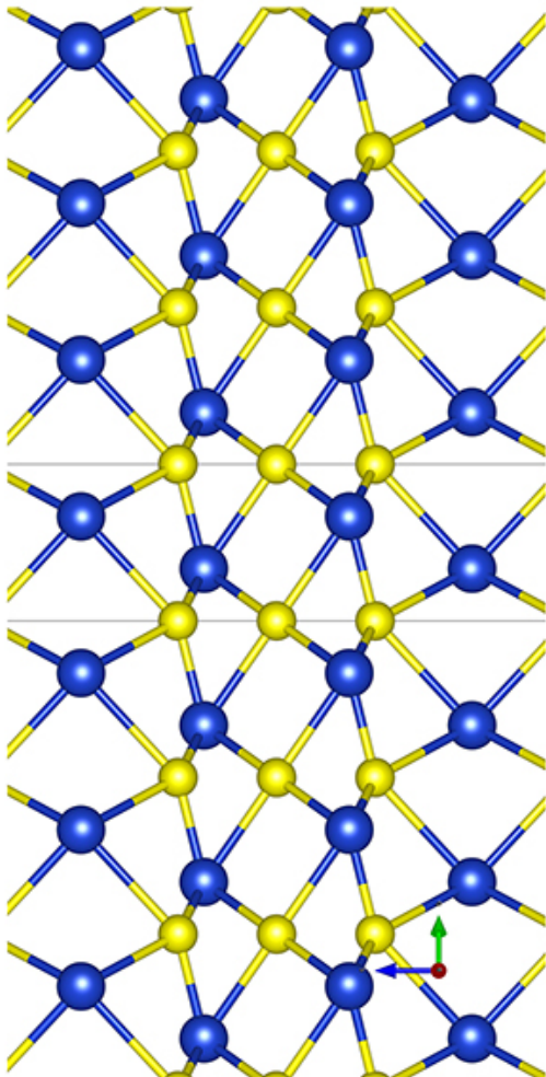
a-Ball&Stick-Mol.jpg
