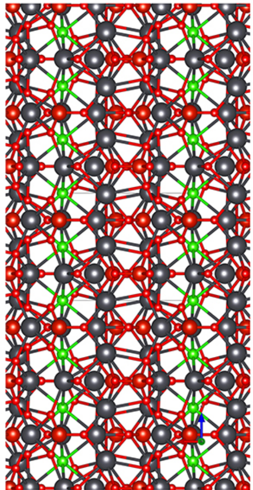
b-Ball&Stick-Mol.jpg
