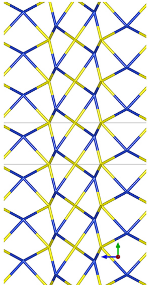
a-Stick-Mol.jpg
