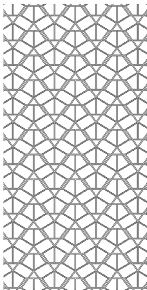
b-Stick-Mol-U.jpg
