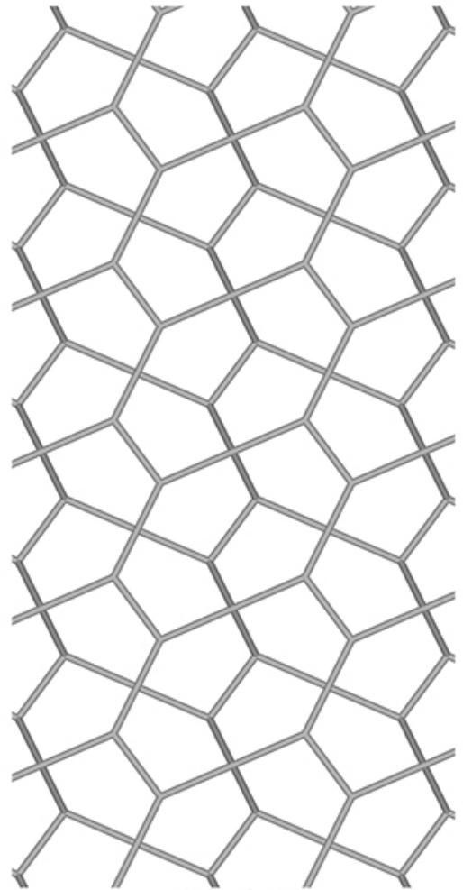
c-Stick-Mol-U.jpg
