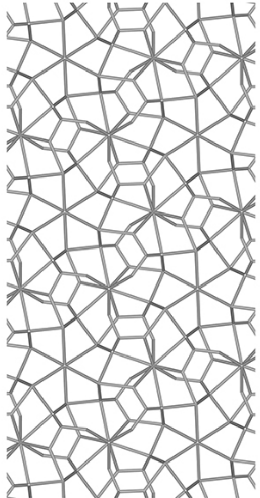
c-Stick-Mol-U.jpg
