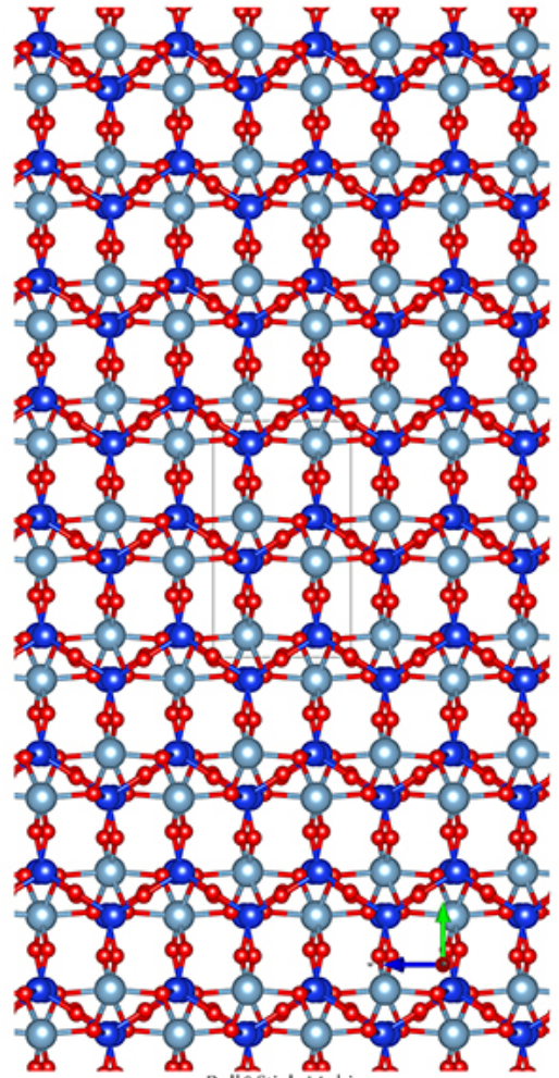
a-Ball&Stick-Mol.jpg
