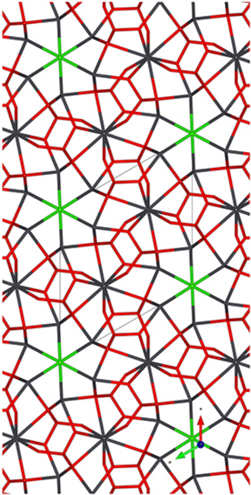
c-Stick-Mol.jpg
