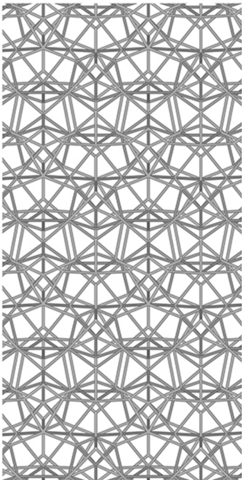
a-Stick-Mol-U.jpg
