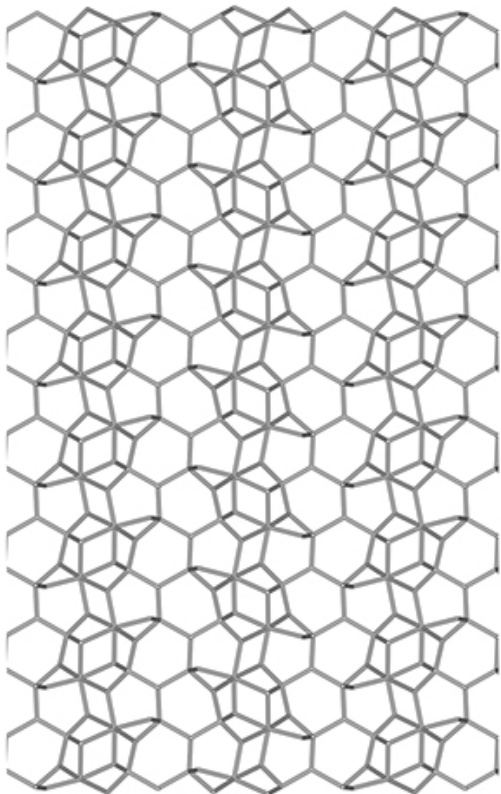
c-Stick-Mol-U.jpg
