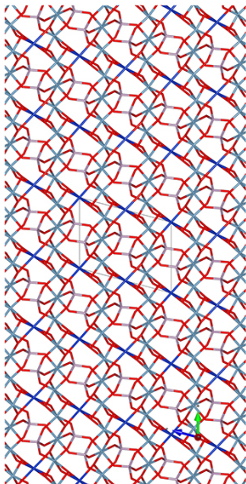
a-Stick-Mol.jpg
