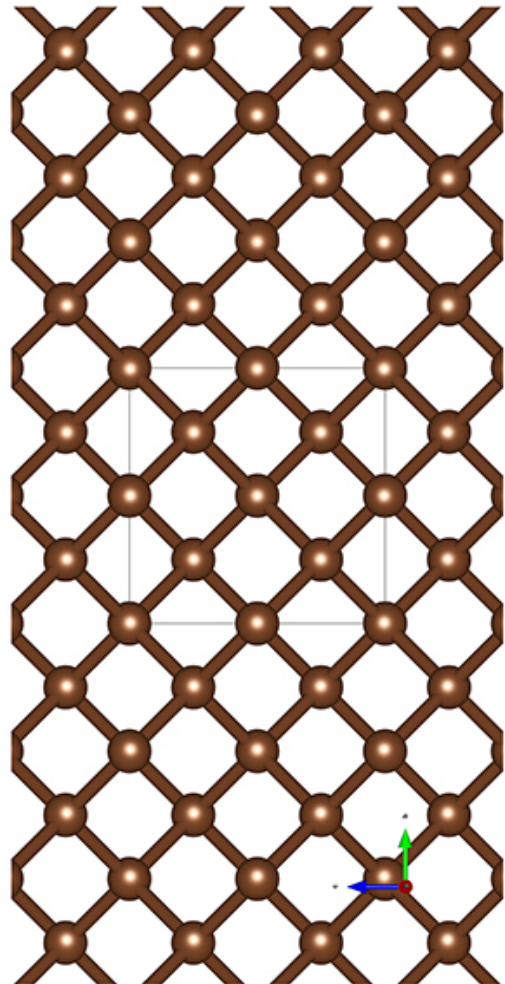
a-Ball&Stick-Mol.jpg
