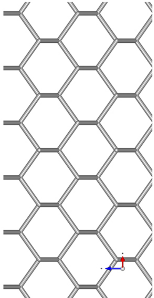
a2-Stick-Mol-U.jpg
