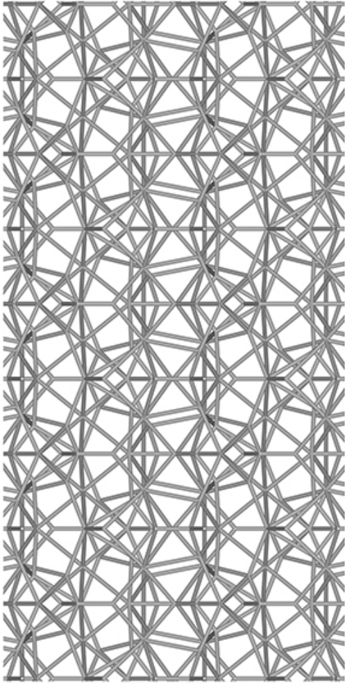
b-Stick-Mol-U.jpg
