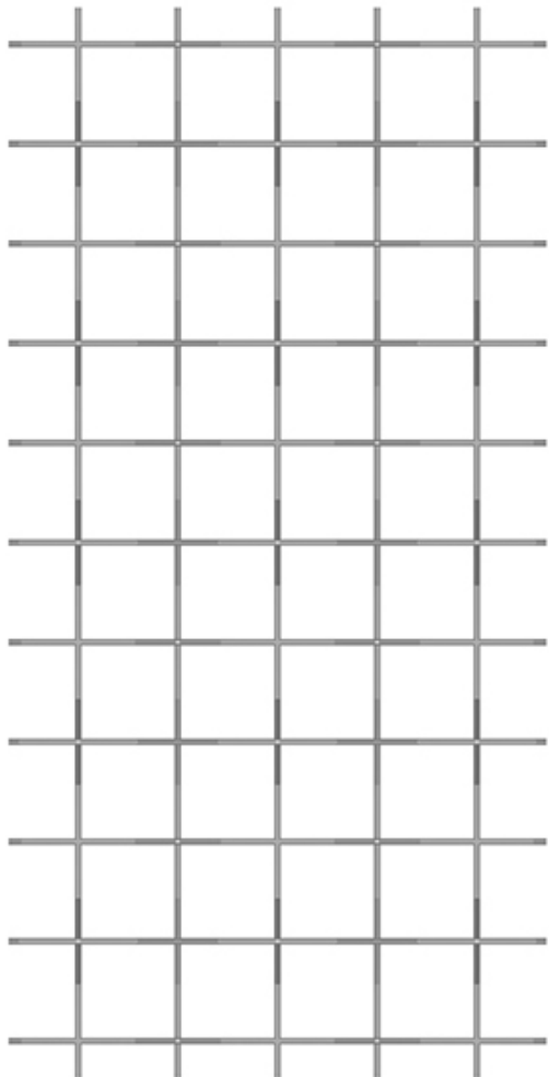
c-Stick-Mol-U.jpg
