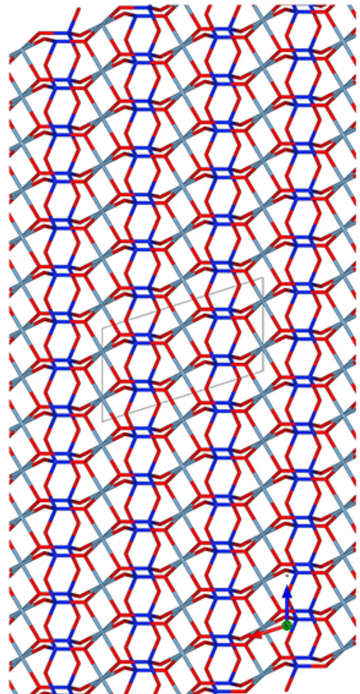
b-Stick-Mol.jpg
