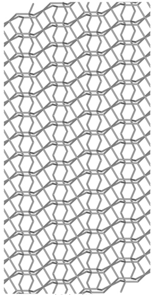
b-Stick-Mol-U.jpg
