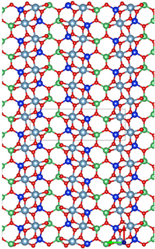
c-Ball&Stick-Mol.jpg
