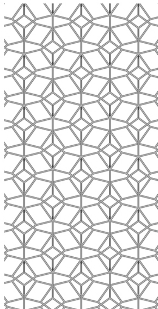
b-Stick-Mol-U.jpg
