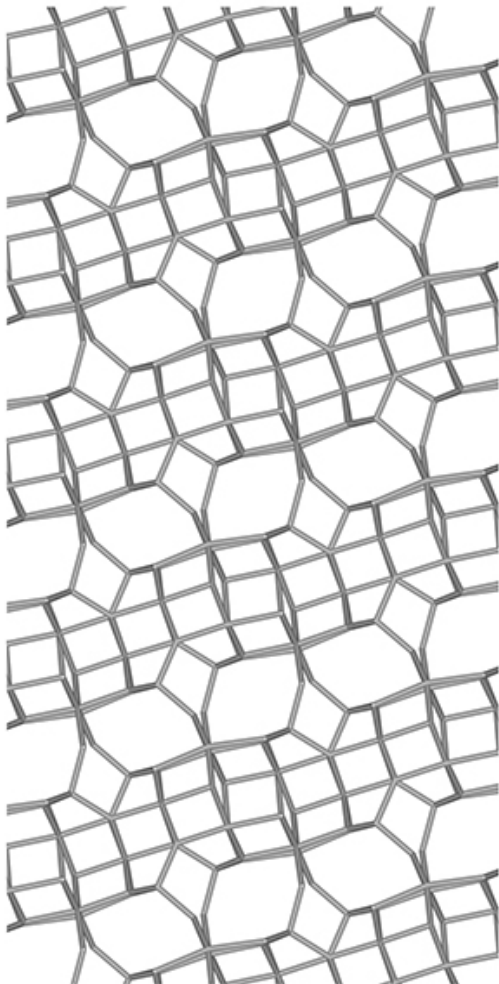
c-Stick-Mol-U.jpg
