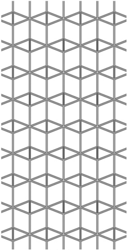
a-Stick-Mol-U.jpg
