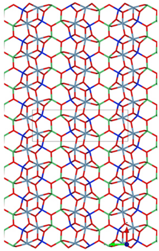
c-Stick-Mol.jpg
