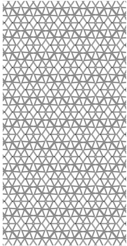
b-Stick-Mol-U.jpg
