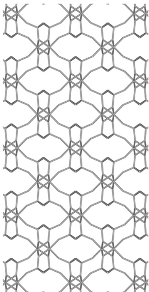
c-Stick-Mol-U.jpg
