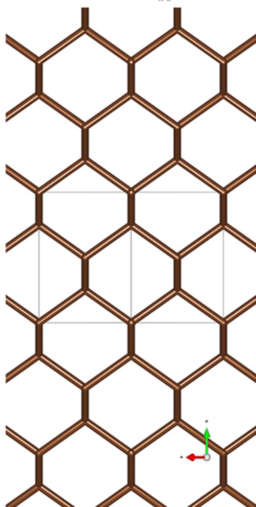
a3-Stick-Mol.jpg
