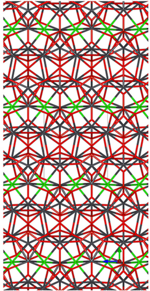
a-Stick-Mol.jpg
