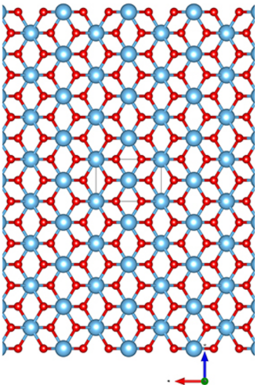
b-Ball&Stick-Mol.jpg
