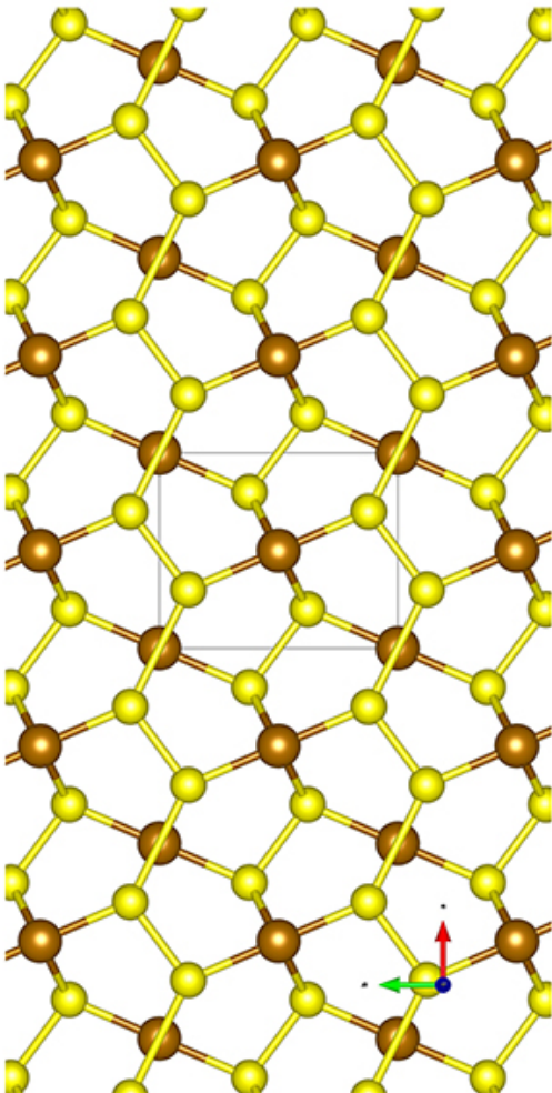
c-Ball&Stick-Mol.jpg
