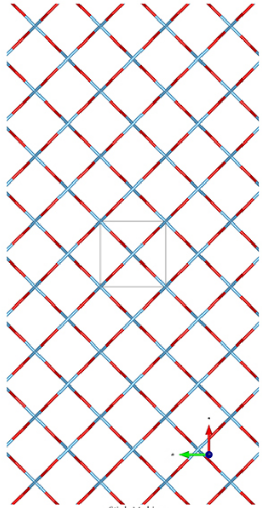
c-Stick-Mol.jpg
