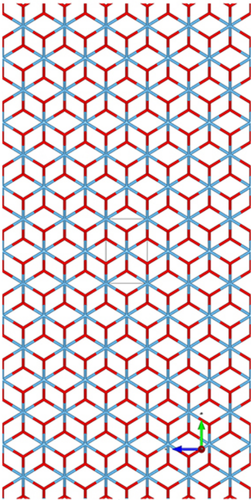
a-Stick-Mol.jpg
