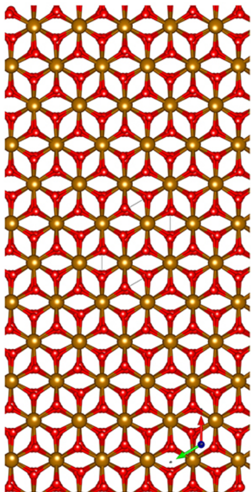
c-Ball&Stick-Mol.jpg
