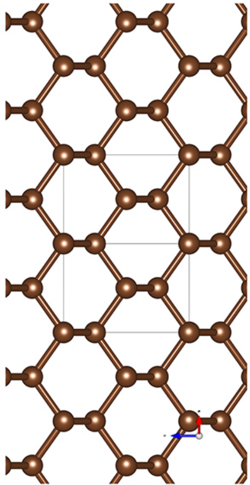
a2-Ball&Stick-Mol.jpg
