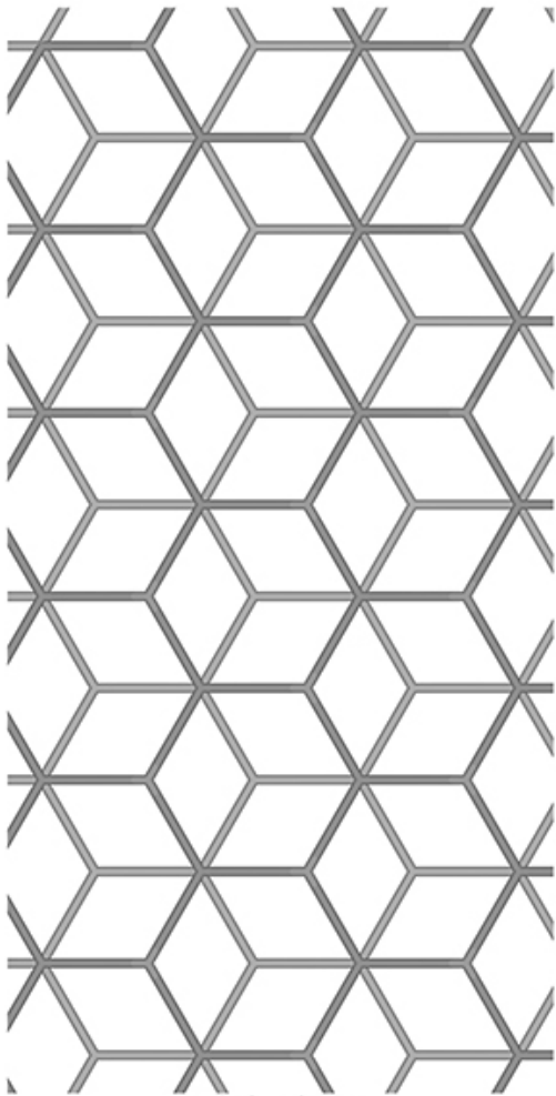
c-Stick-Mol-U.jpg
