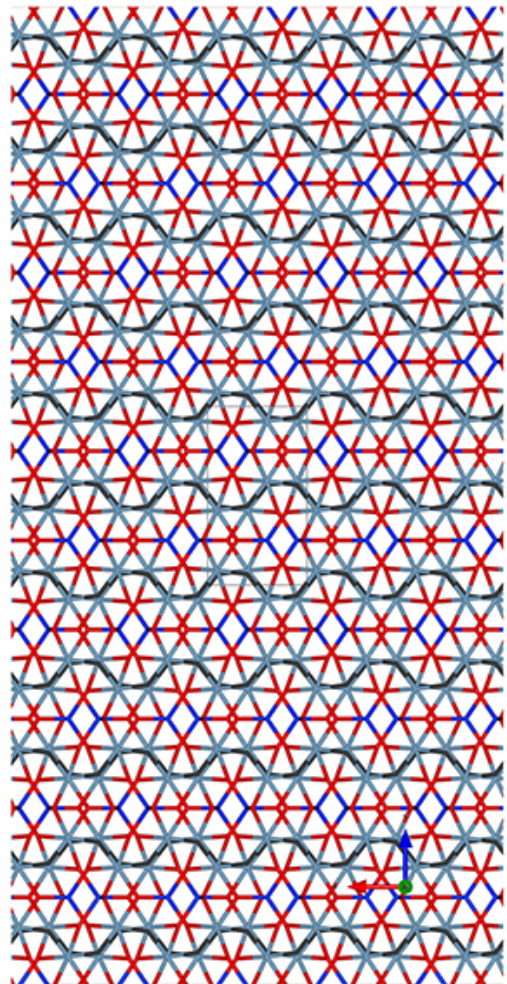
b-Stick-Mol.jpg
