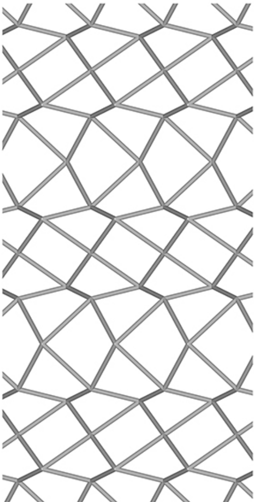
b-Stick-Mol-U.jpg
