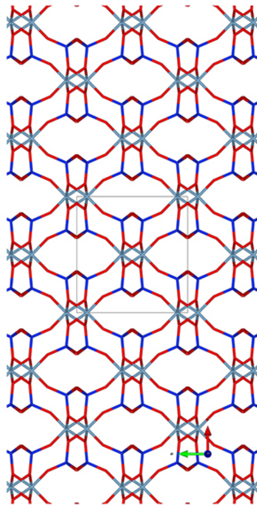
c-Stick-Mol.jpg
