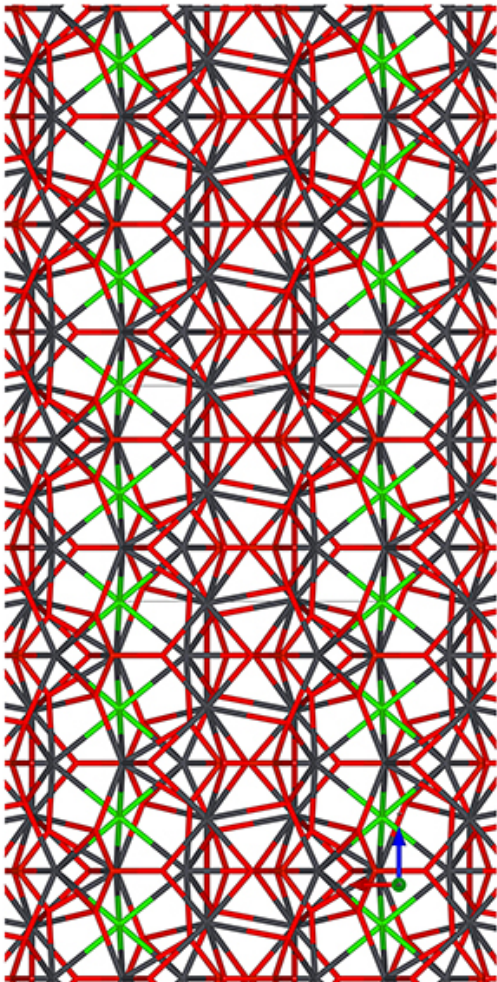
b-Stick-Mol.jpg
