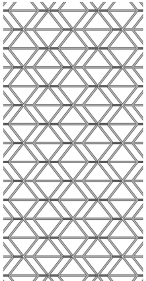
b-Stick-Mol-U.jpg
