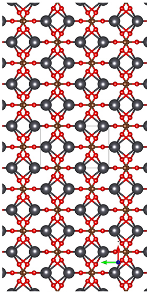
c-Ball&Stick-Mol.jpg
