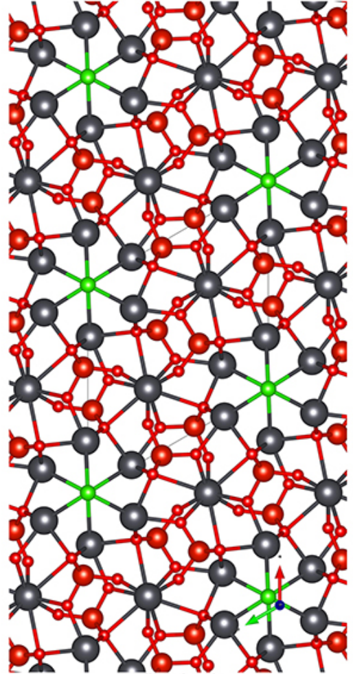
c-Ball&Stick-Mol.jpg
