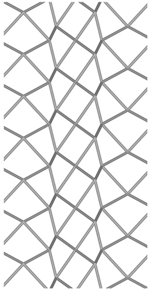
a-Stick-Mol-U.jpg
