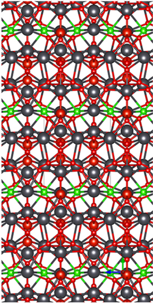
a-Ball&Stick-Mol.jpg
