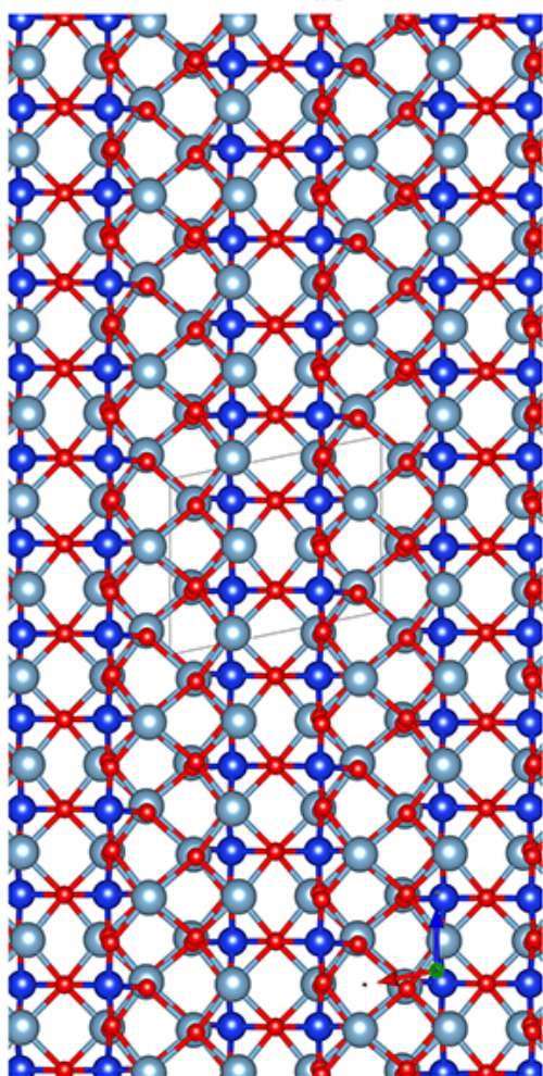
b-Ball&Stick-Mol.jpg
