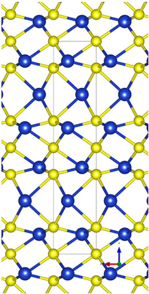
b-Ball&Stick-Mol.jpg
