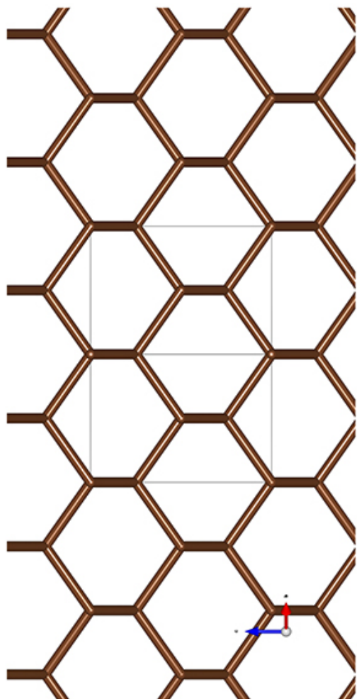
a2-Stick-Mol.jpg
