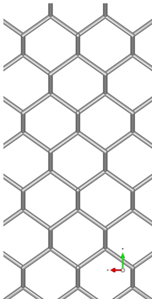
a3-Stick-Mol-U.jpg
