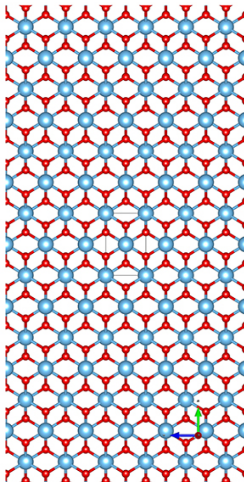
a-Ball&Stick-Mol.jpg
