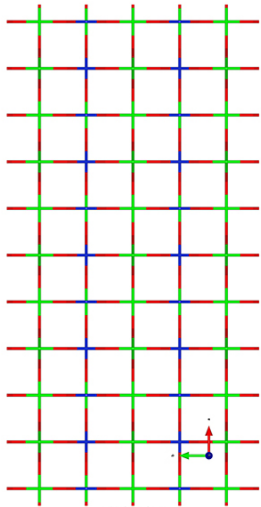
c-Stick-Mol.jpg
