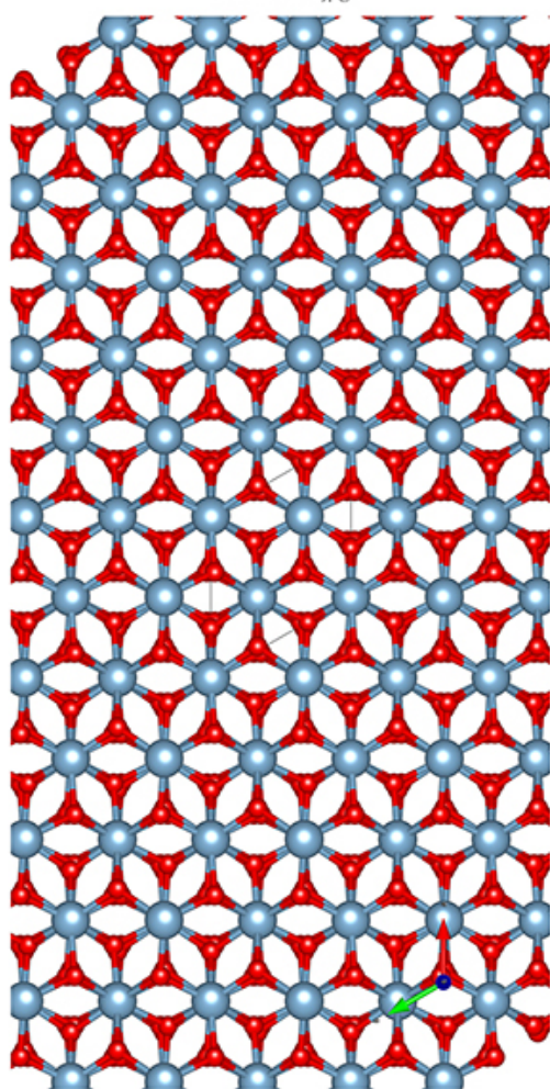
c-Ball&Stick-Mol.jpg
